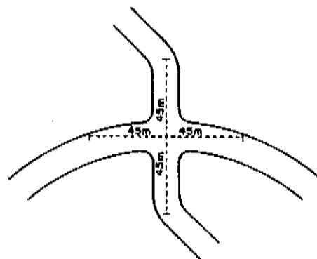
INTERSECTION ET CHAMP DE VISIBILITÉ
