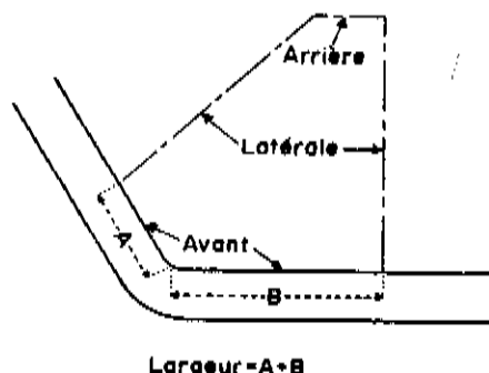
LARGEUR D'UN LOT D'ANGLE
