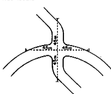
INTERSECTION ET CHAMP DE VISIBILITÉ
