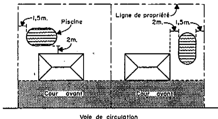
IMPLANTATION D'UNE PISCINE CREUSÉE
