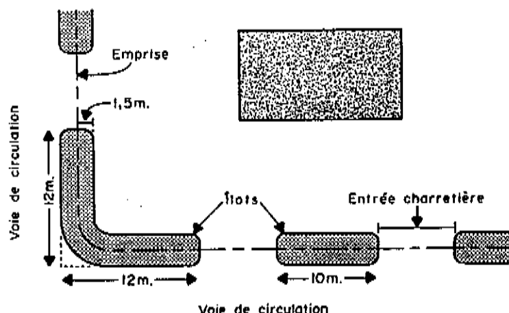
LOCALISATION DES ENTRÉES CHARRETIÈRES
