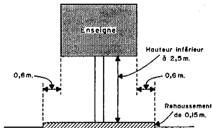
CERCLE DE PROTECTION
