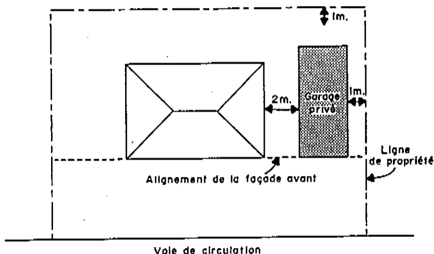
IMPLANTATION D'UN GARAGE PRIVÉ
