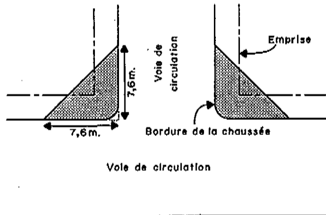
TRIANGLE DE VISIBILITÉ
