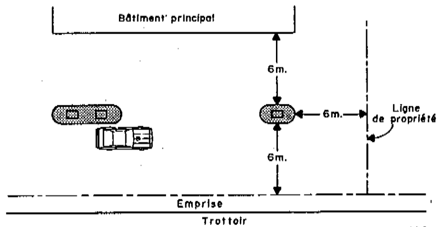
IMPLANTATION DES UNITÉS DE DISTRIBUTION D'ESSENCE (POMPES)
