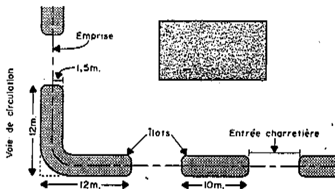
LOCALISATION DES ENTRÉES CHARRETIÈRES
