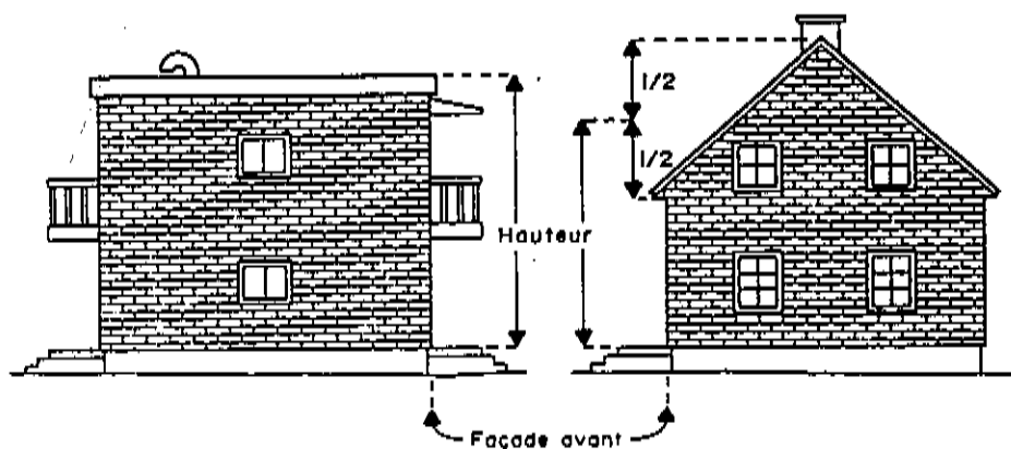
HAUTEUR D'UN BÂTIMENT EN MÈTRE
