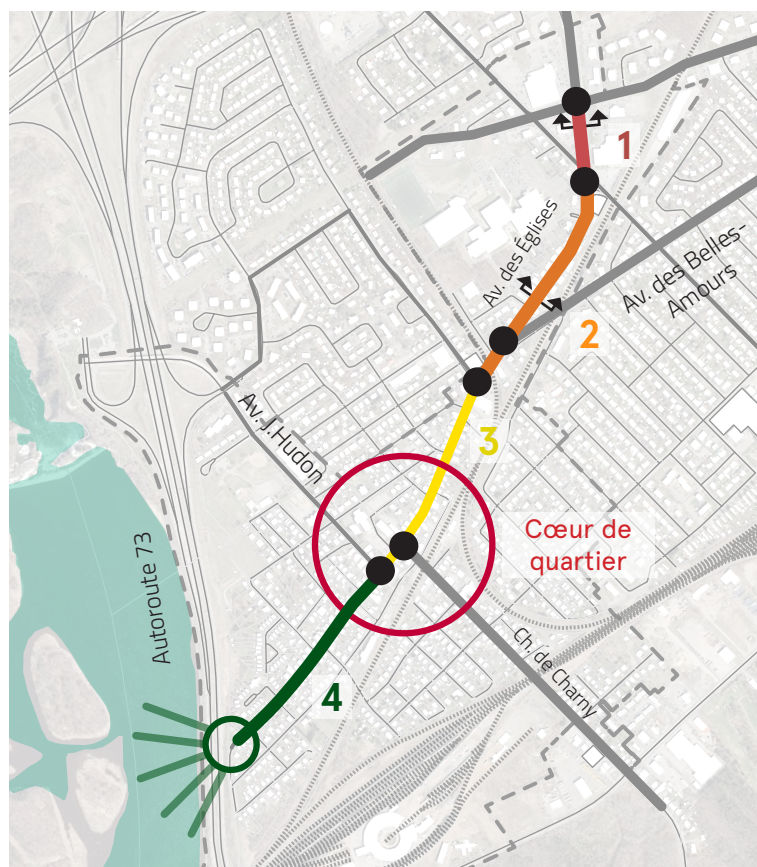
Figure 55 : Localisation des tronçons de l'Avenue des Églises — Localisation des profils schématiques
