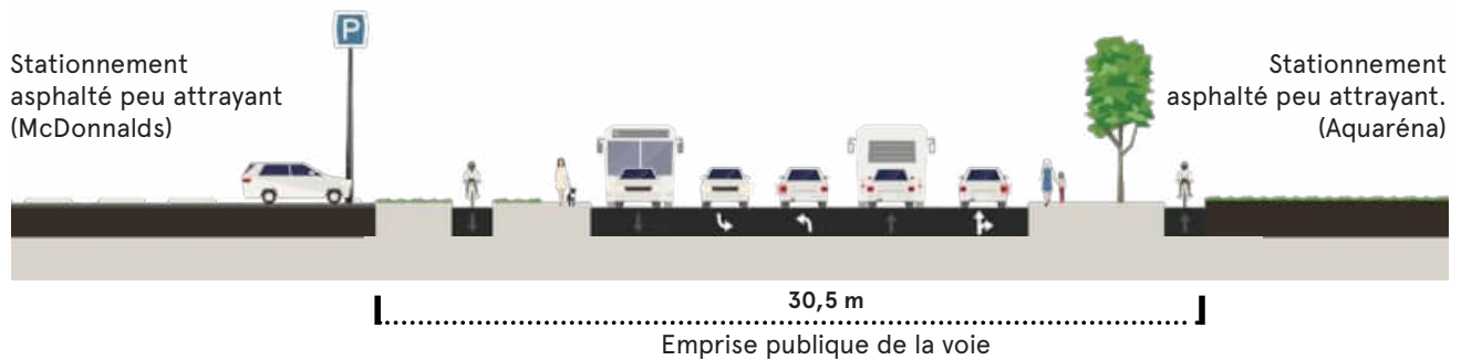
Figure 57 : Vision du réaménagement des tronçons de l'Avenue des Églises
