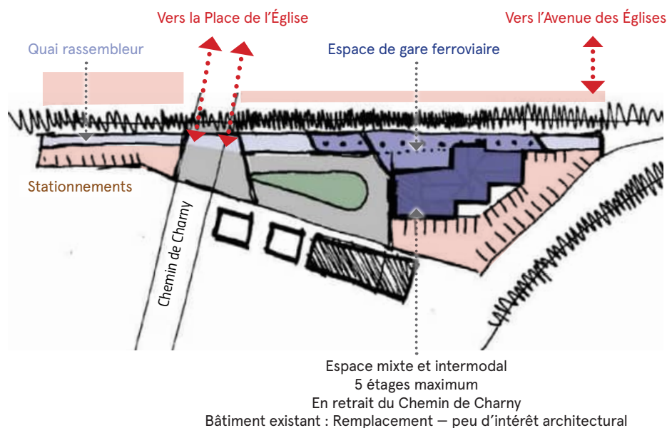
Figure 52 : Exemple de schéma de principe d'aménagement pour le secteur de la gare
